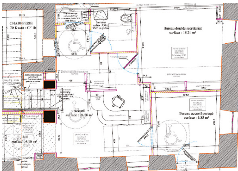
Plan de l'accueil du rez de chaussée
